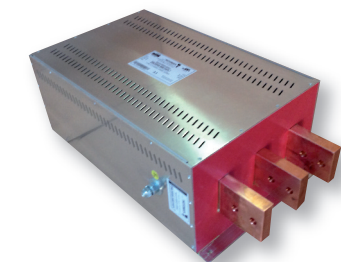
FIN1500.(1750 - 3000).BC
